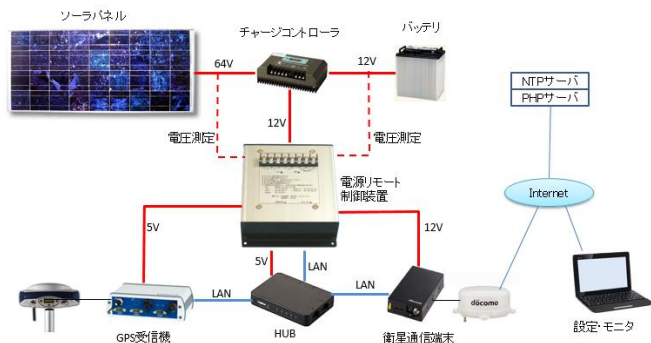
活火山観測装置用電源制御装置
